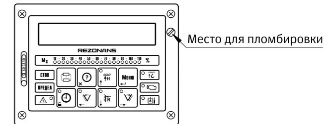
Рисунок 15. Пломбирование прибора безопасности
