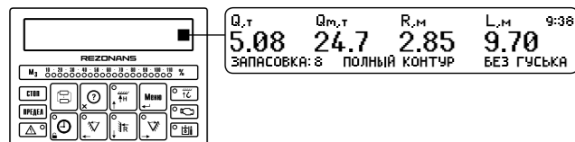
Рисунок 6. Основные параметры крана
