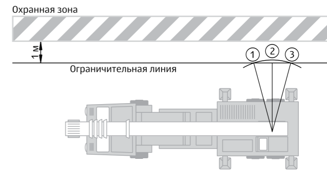
Рисунок 11. Координатная защита «Стена»
