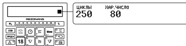
Рисунок 9. Долговременная информация о состоянии крана
