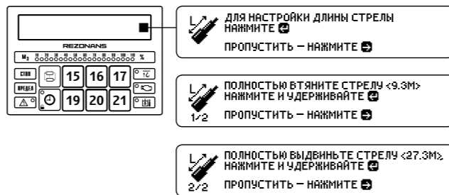
Рисунок 20. Задание коэффициентов для определения длины стрелы
