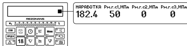
Рисунок 8. Диагностическая информация о состоянии крана
