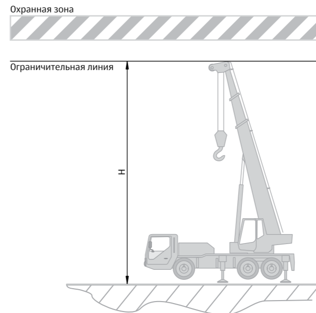
Рисунок 10. Координатная защита «Потолок»
