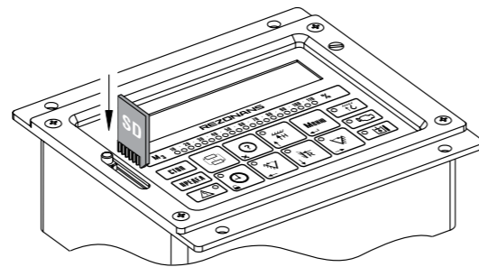
Рисунок 13. Разъем для SD-карты в блоке индикации
