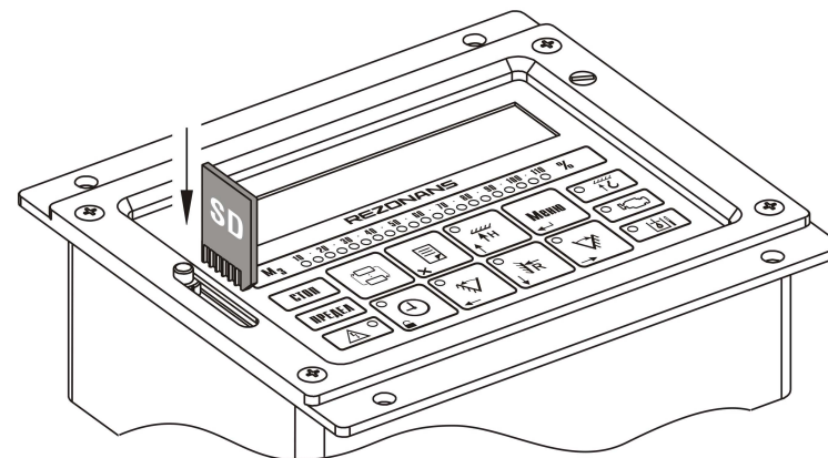
Р и с у н о к 14 — Разъем для SD-карты в блоке индикации
