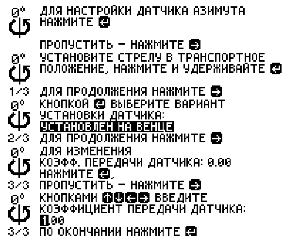
Рисунок 23 — Установка начала отсчета датчика азимута
