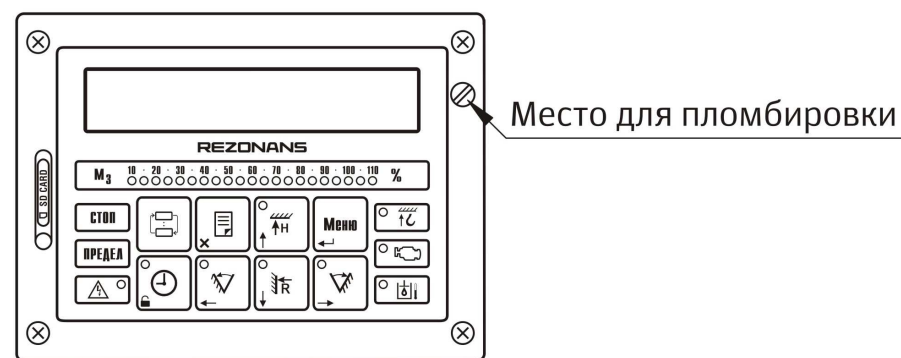
Р и с у н о к 17 — Пломбирование прибора безопасности
