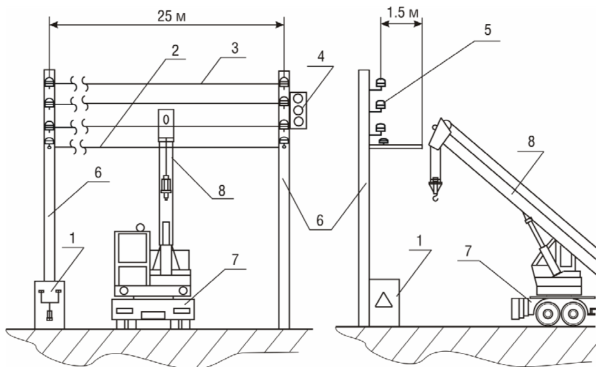
1 – щиток ЛЭП; 2 – капроновый канат; 3 – проводники макета ЛЭП; 4 – светильники; 5 – изоляторы; 6 – опоры проводников макета ЛЭП; 7 – грузоподъемный кран; 8 – стрела крана.
