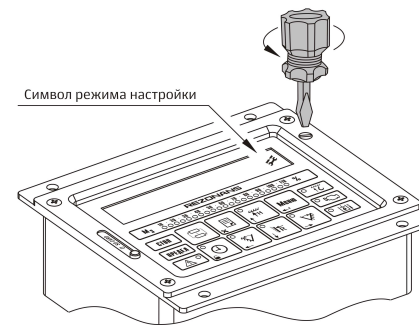
Рисунок 18 — Переключатель режима настройки
