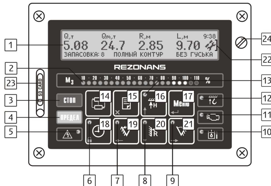
Рисунок 2 — Лицевая панель блока индикации БИ04
