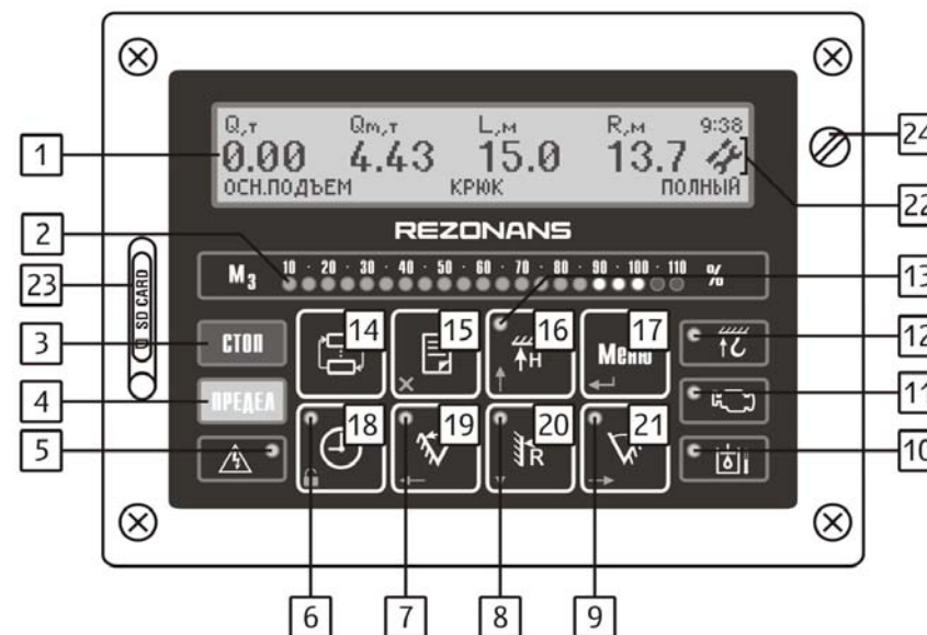
Рисунок 2 — Лицевая панель блока индикации БИ04
