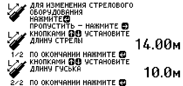
Рисунок 19 — Выбор длины стрелы и гуська
