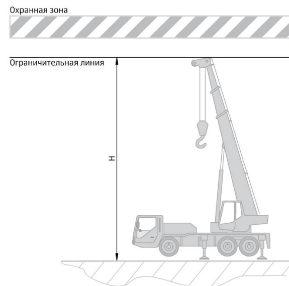
Рисунок 10 — Координатная защита «Потолок»
