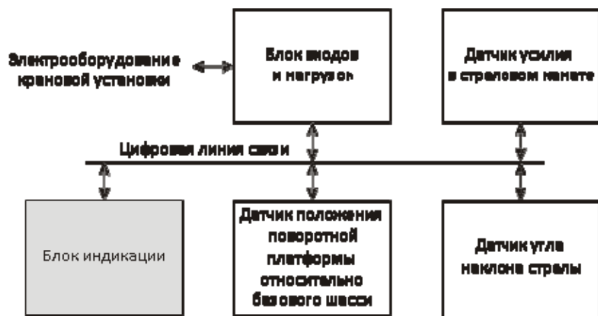
Рисунок 1 — Структурная схема ОГМ240
