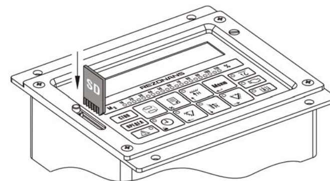
Р и с у н о к 13 — Разъем для SD-карты в блоке индикации
