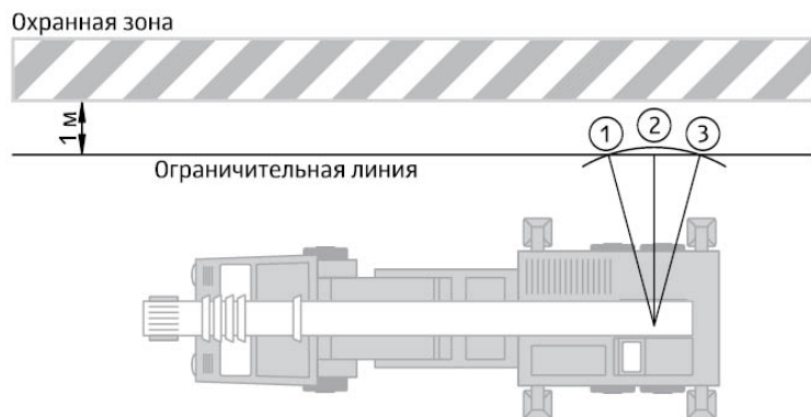
Рисунок 11 — Координатная защита «Стена»
