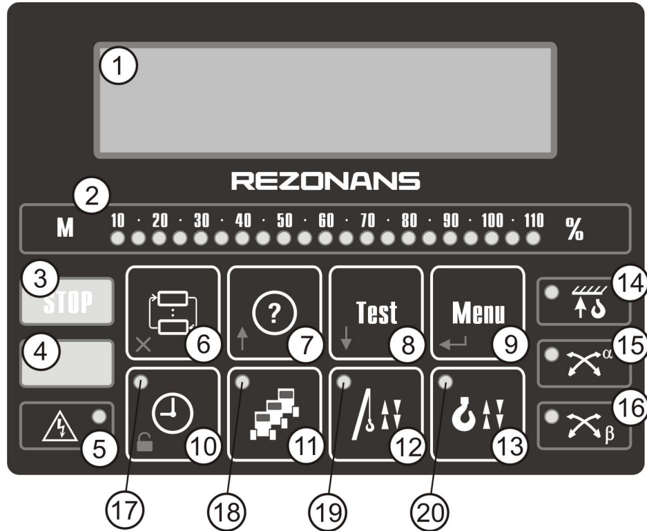
Рисунок 1 — Лицевая панель блока индикации БИ04.11
