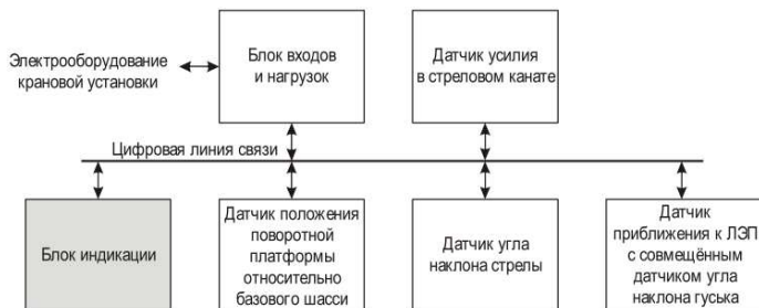
Рисунок 1 — Структурная схема ОГМ240
