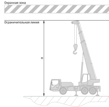
Рисунок 10 — Координатная защита «Потолок»
