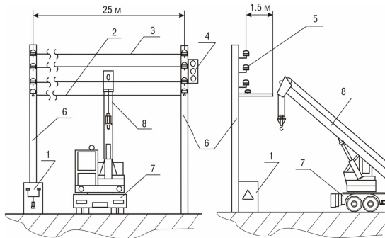
Рисунок 13 — Макет линии электропередач
