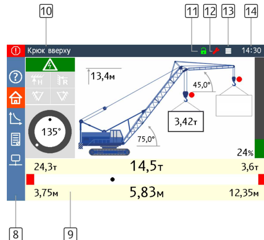
Рисунок 3 — Графический интерфейс блока индикации БИ04.70
