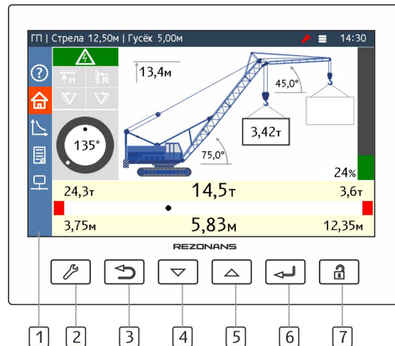
Рисунок 2 — Лицевая панель блока индикации БИ04.70
