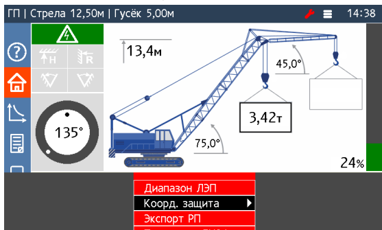
Рисунок 9 — Меню блока индикации
