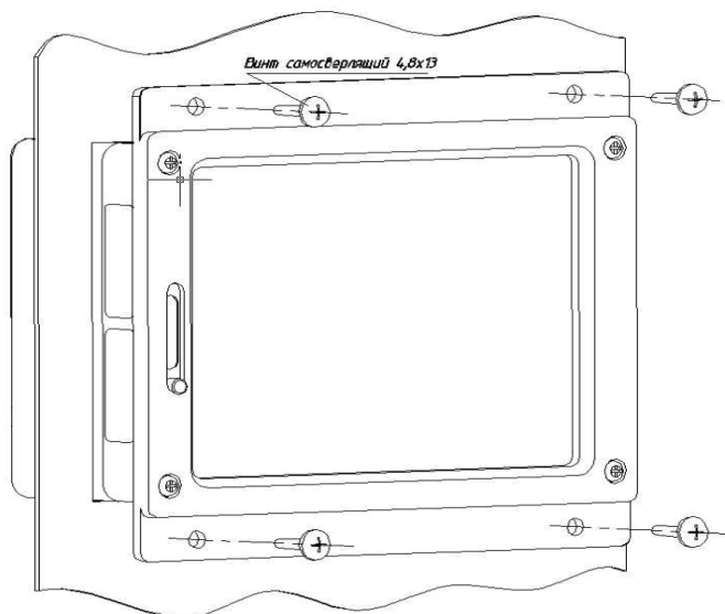
Рисунок 2 — Установка БИ04.43-0
