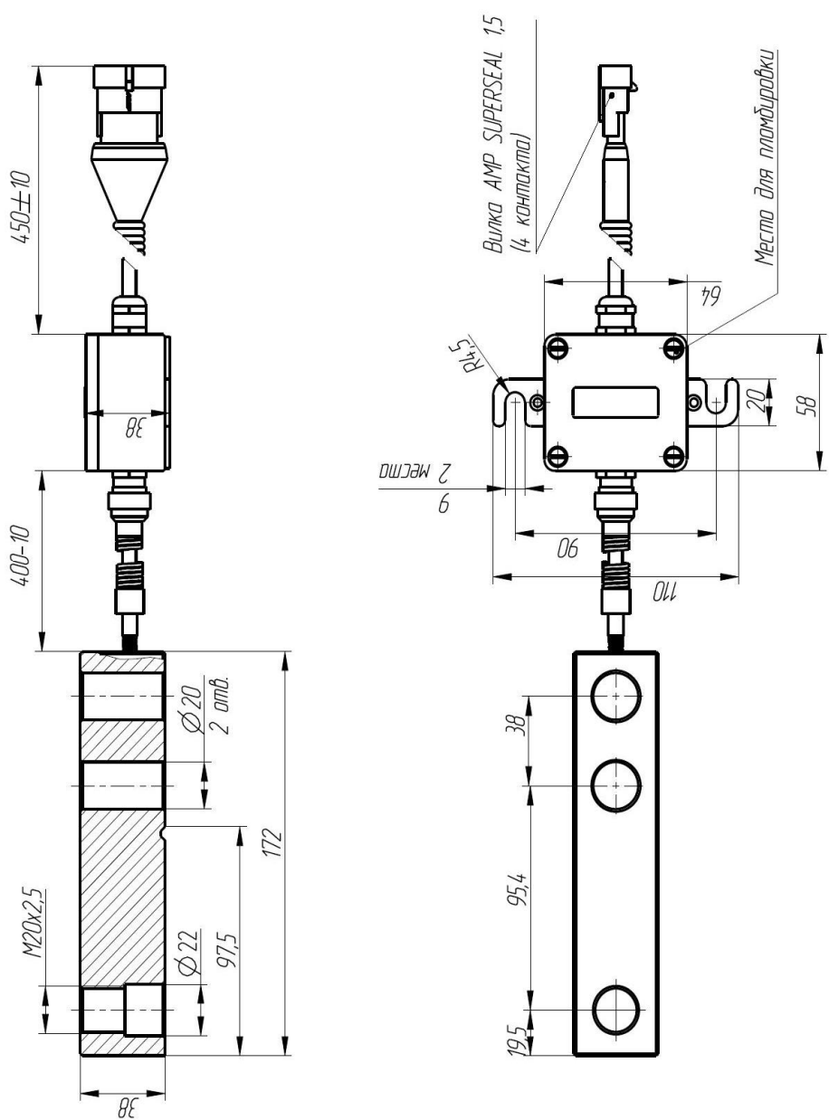
Рисунок 16 — Габаритные и присоединительные размеры датчика усилия балочного типа серии ТКС-5000-Р114-Х
