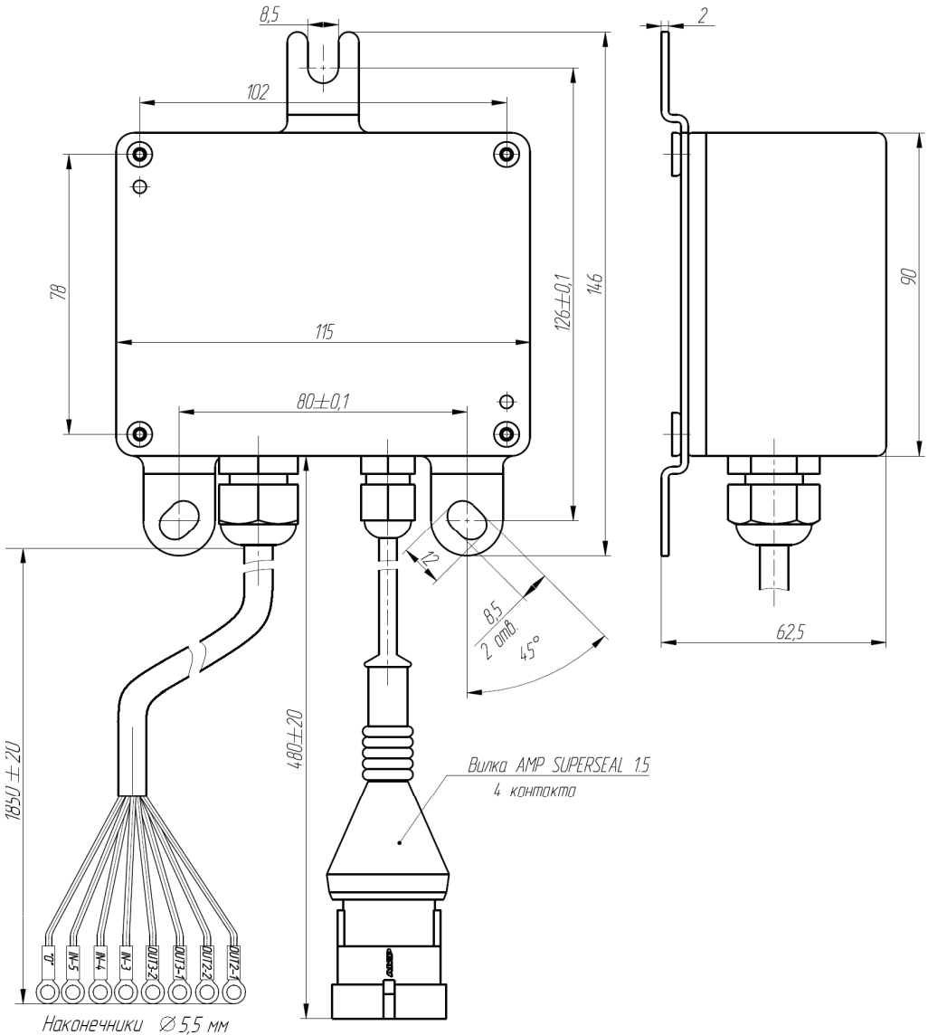
Рисунок 10 — Габаритные и присоединительные размеры БВН2.4
