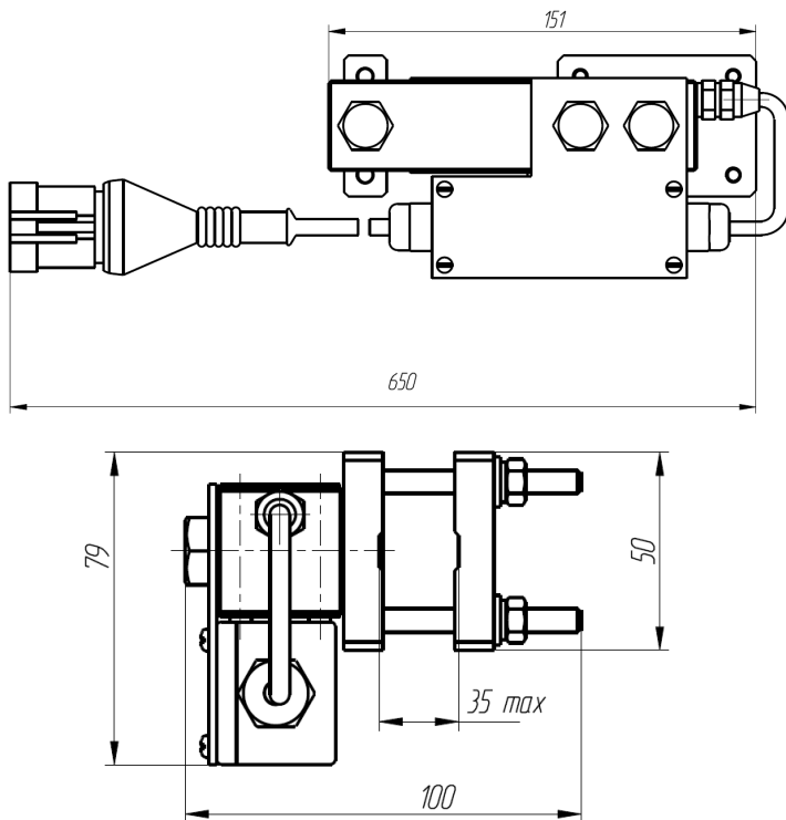
Рисунок 14 — Габаритные и присоединительные размеры датчика усилия на канат (изгиба) серии ТКС
