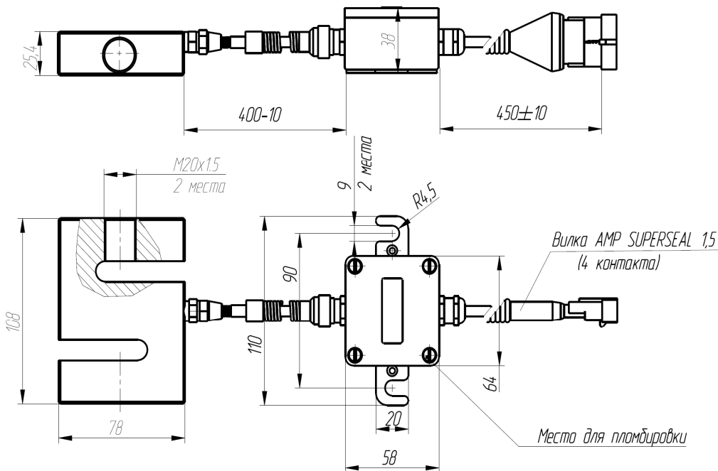
Рисунок 11 — Габаритные и присоединительные размеры датчика усилия сжатия серии ТСС-5000-Р113-Х
