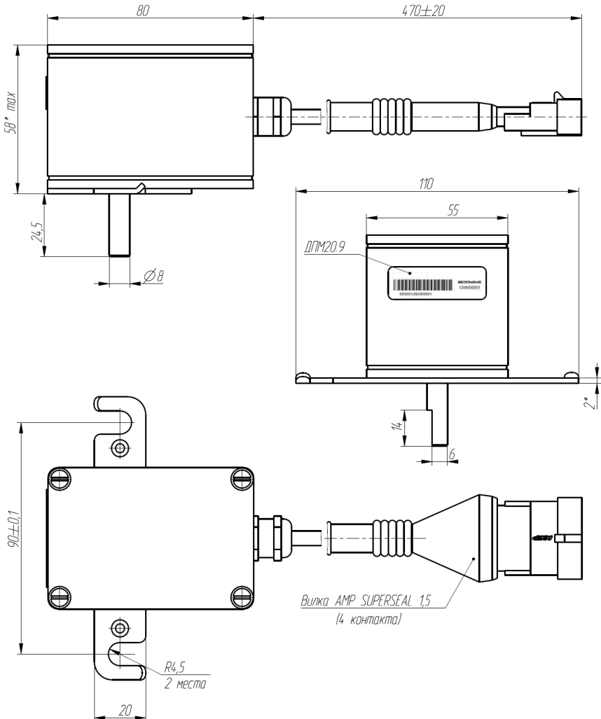
Рисунок 8 — Габаритные и присоединительные размеры датчика серии ДПМ20.9
