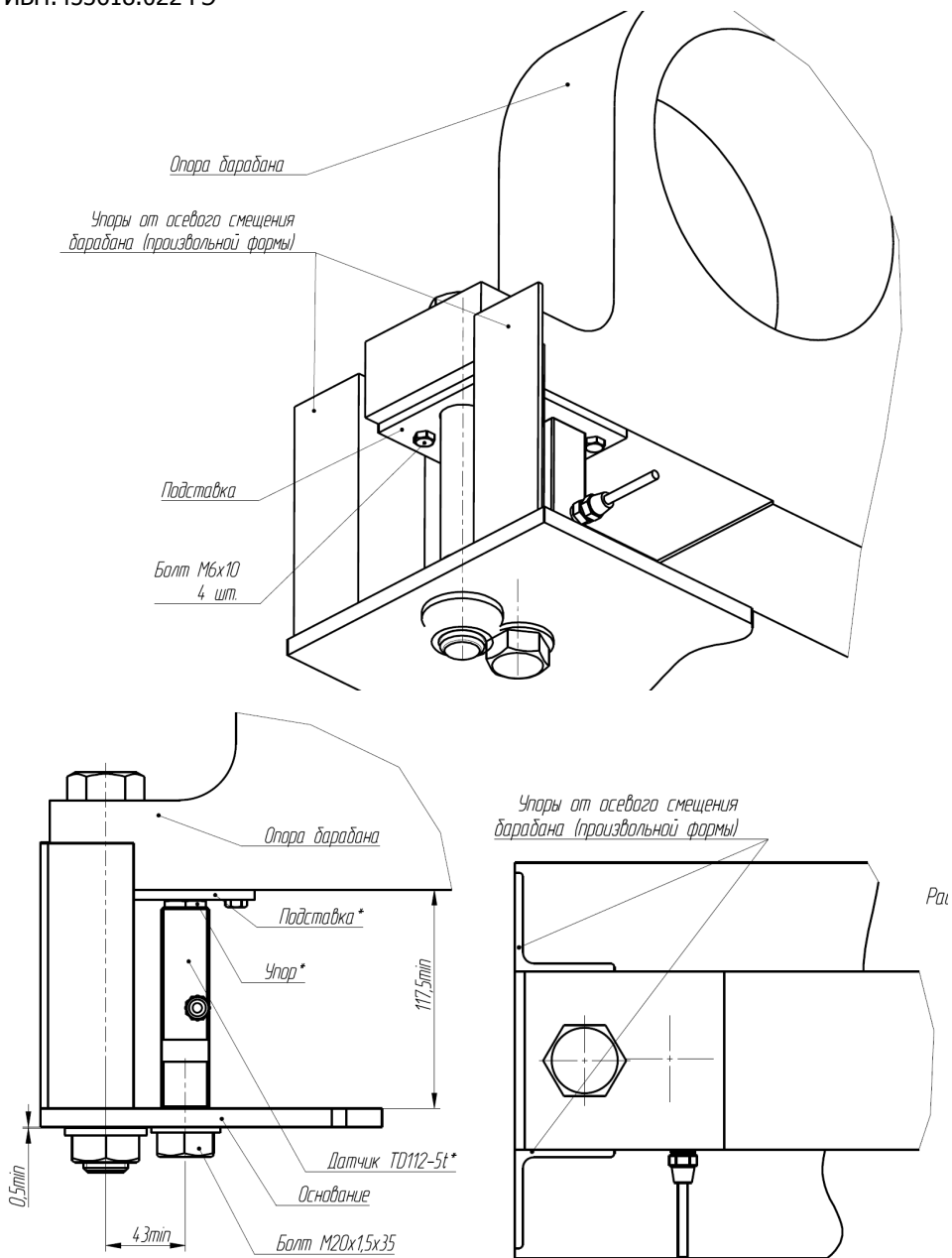
Рисунок 13 — Пример установки датчиков серии ТСС-5000-Р113-Х
