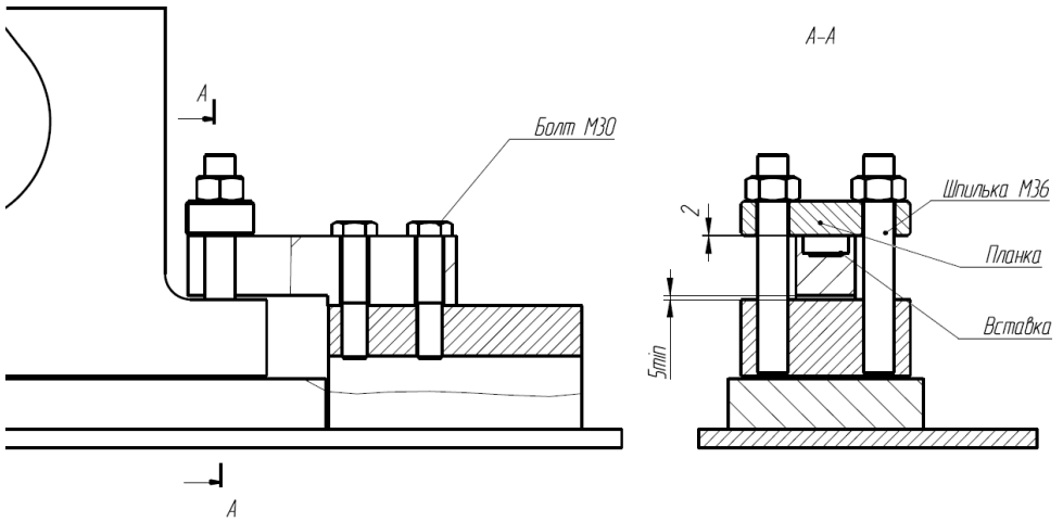
Рисунок 19 — Пример установки датчика усилия балочного типа серии ТКС для опоры барабана
