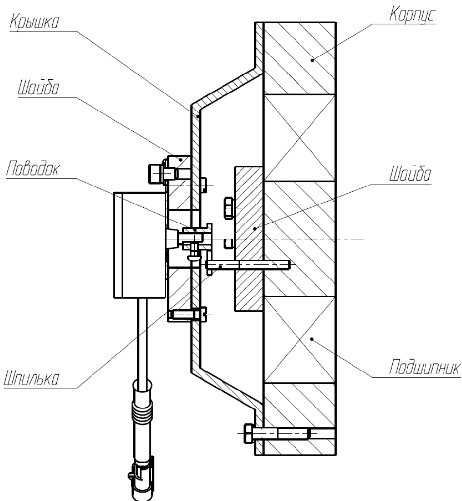
Рисунок 9 — Пример установки датчика угла поворота на барабан лебёдки для отслеживания осевого вращения.
