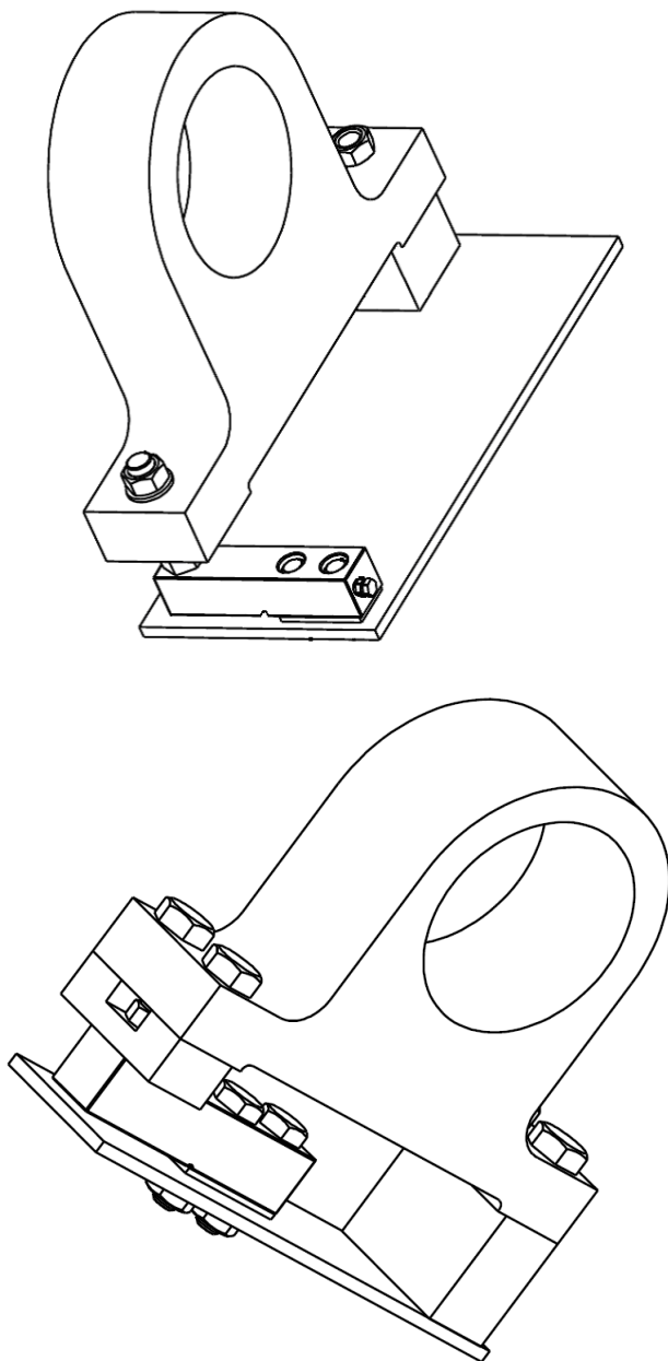
Рисунок 23 — Примеры установки датчиков усилия балочного типа серии ТКС под опору барабана
