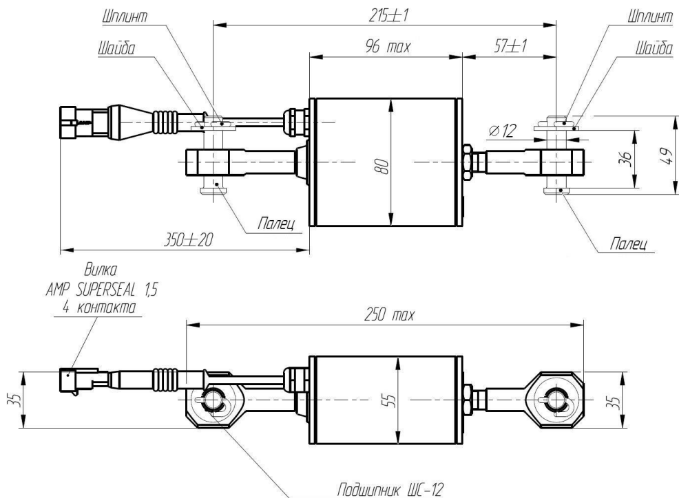
Рисунок 26 — Габаритные и присоединительные размеры датчика усилия растяжения серии ТРС-1000-Р111-Х
