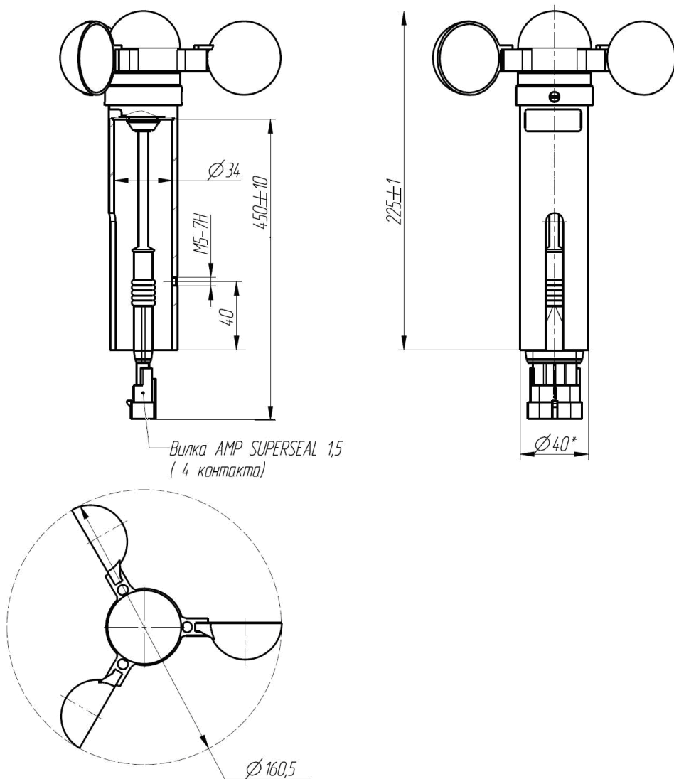
Рисунок 7 — Габаритные и присоединительные размеры ДСВ1.13 и МС1-Р11
