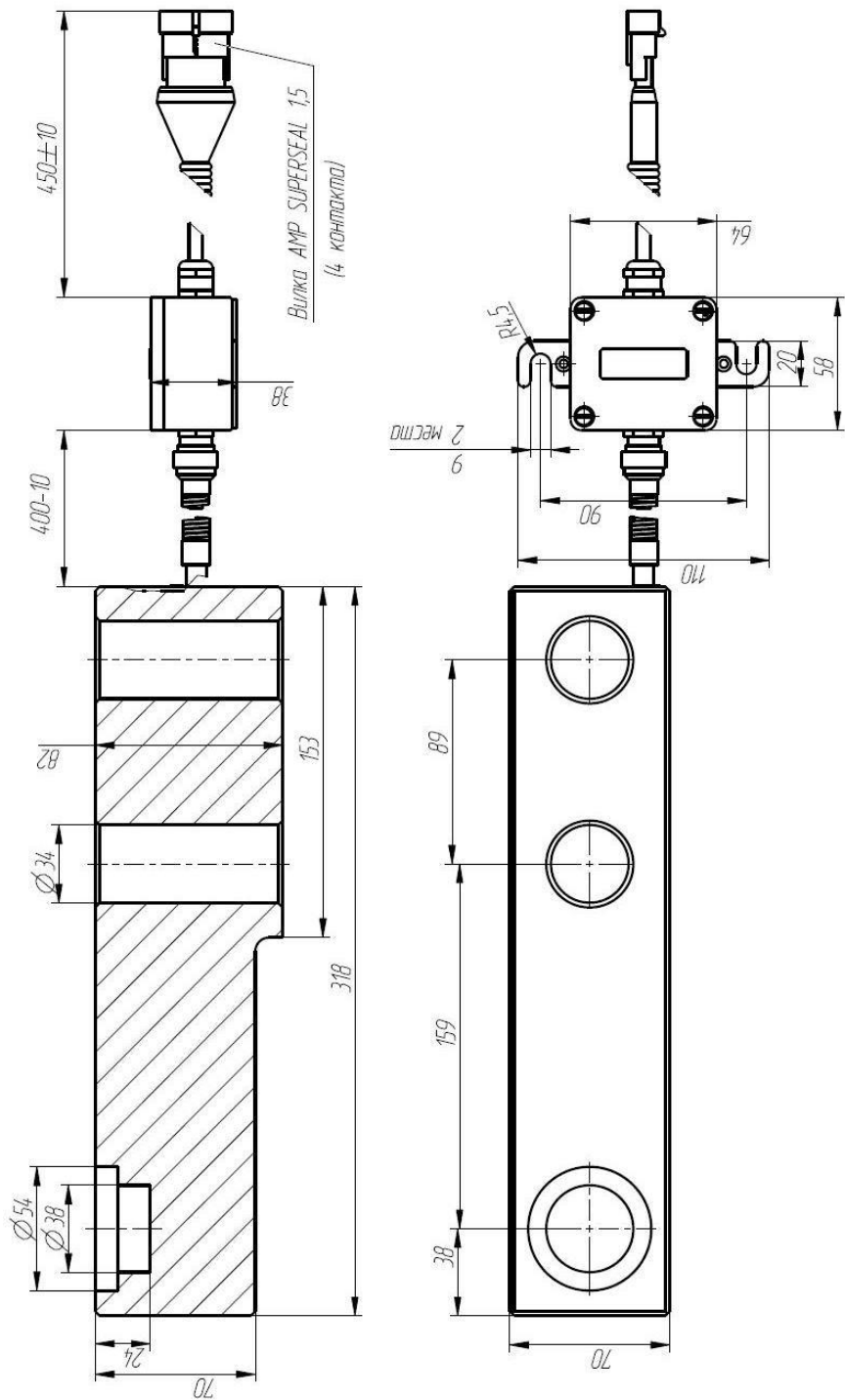
Рисунок 18 — Габаритные и присоединительные размеры датчика усиления балочного типа серии ТКС-20000-Р115-1
