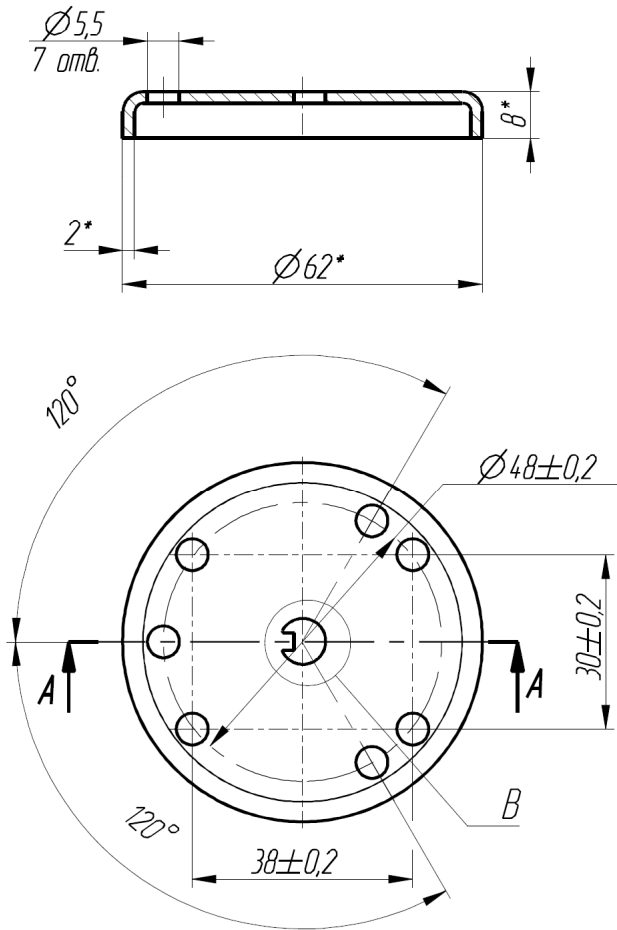
Рисунок 6 — Габаритные и присоединительные размеры сферы для крепления БИ04.43-1
