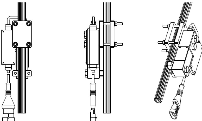
Рисунок 15 — Пример установки датчиков серии ТКС на канат
