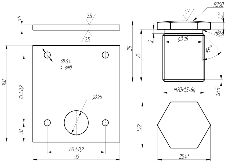
Прокладка РИВП.741434.005
