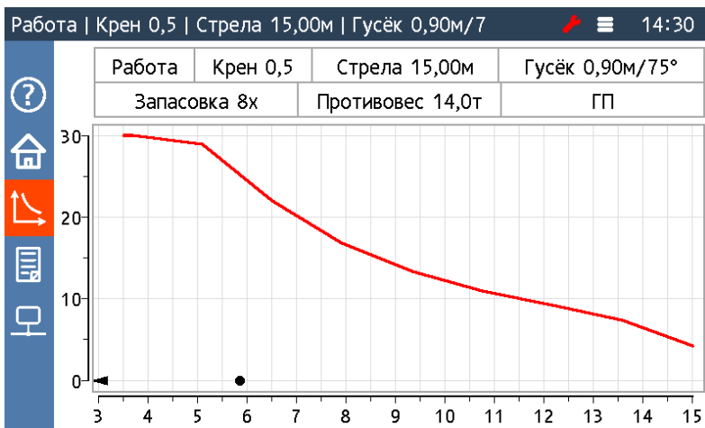
Рисунок 6 — Экран грузовой характеристики
