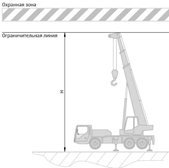
Рисунок 10 — Координатная защита «Потолок»
