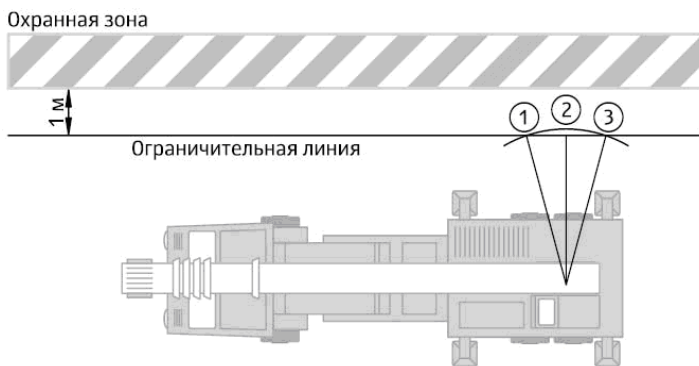
Рисунок 11 — Координатная защита «Стена»
