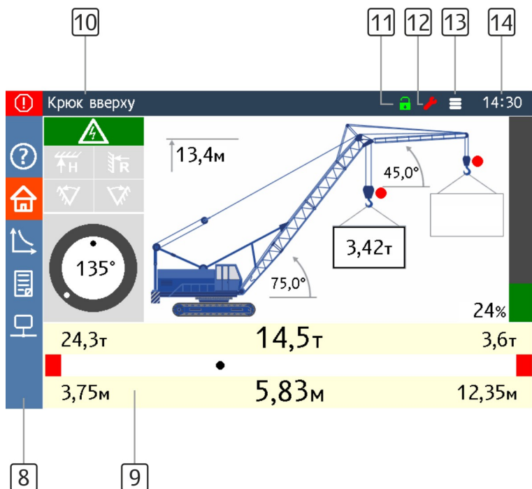
Рисунок 3 — Графический интерфейс блока индикации БИ04.70
