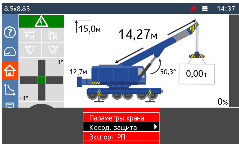
Рисунок 10 — Меню блока индикации
