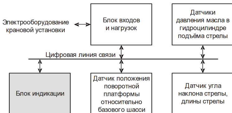
Рисунок 1 — Структурная схема ОГМ240
